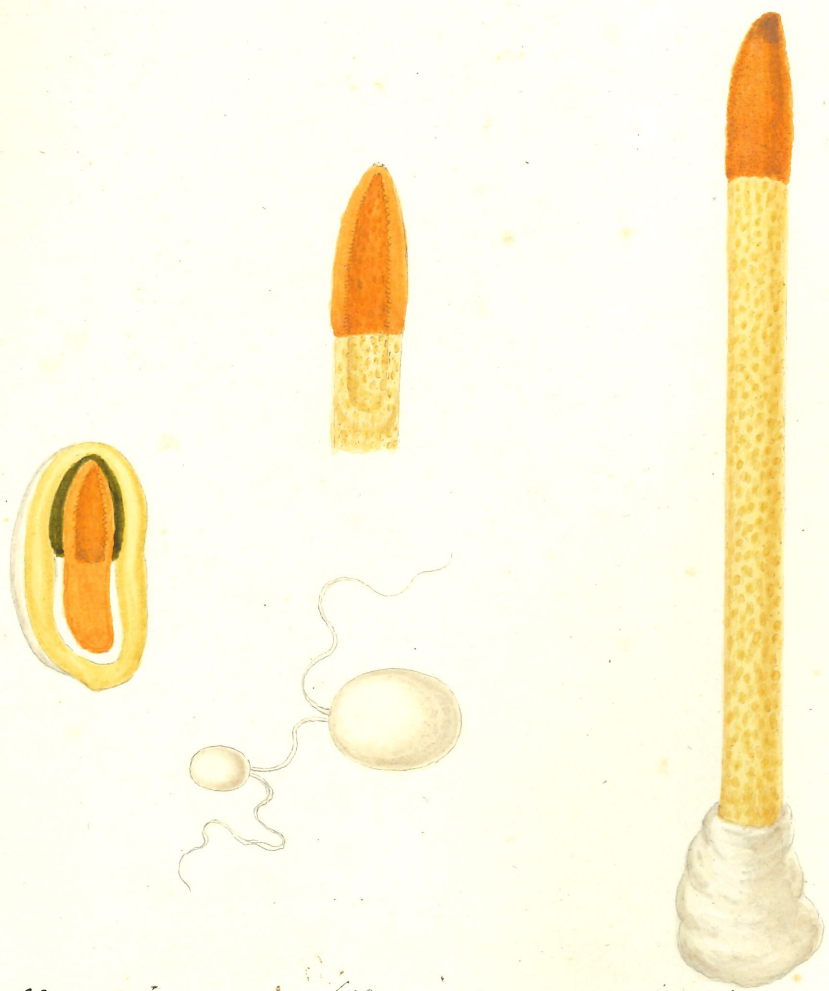
Mutinus caninus . (Phallus, Huds.)
